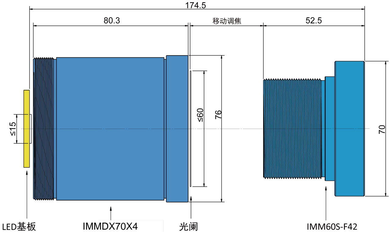
图 2：高清成像投影光路示意图
