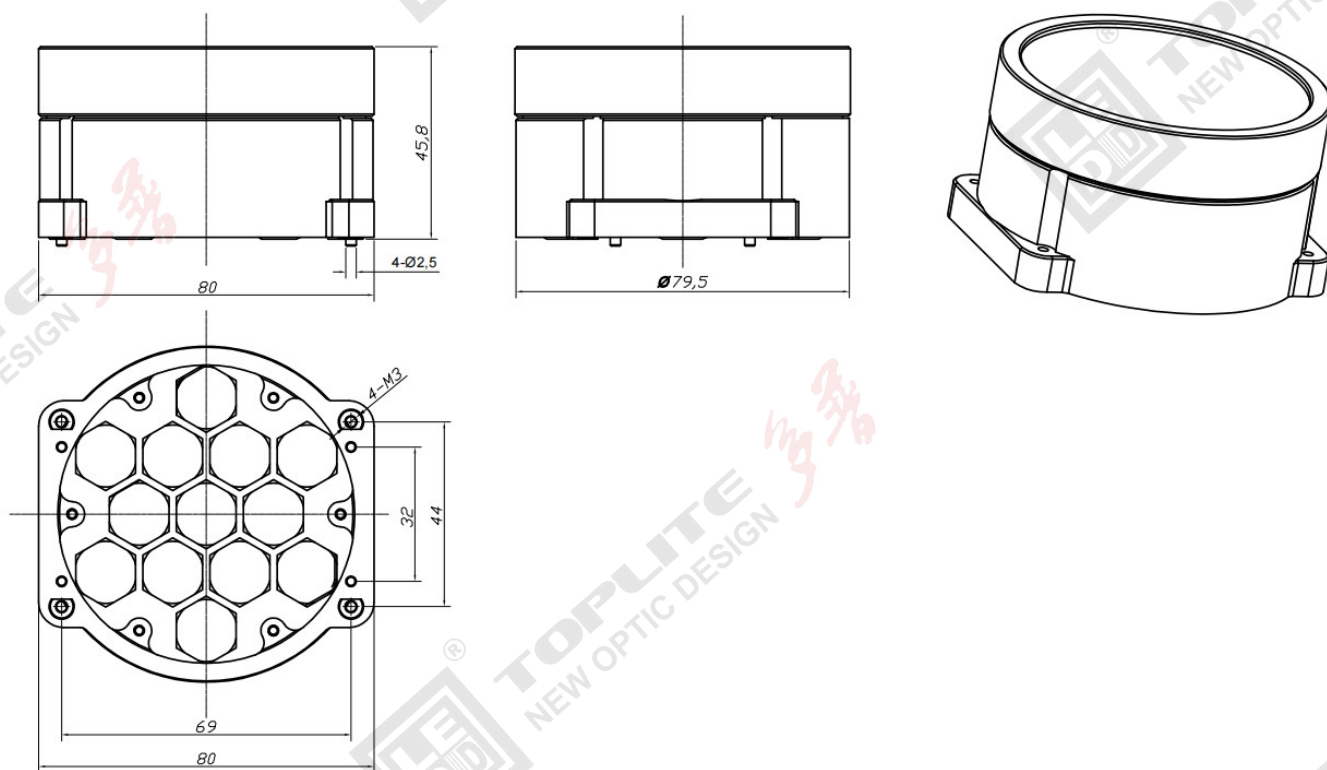
图 2：激光模组光学件外形尺寸
