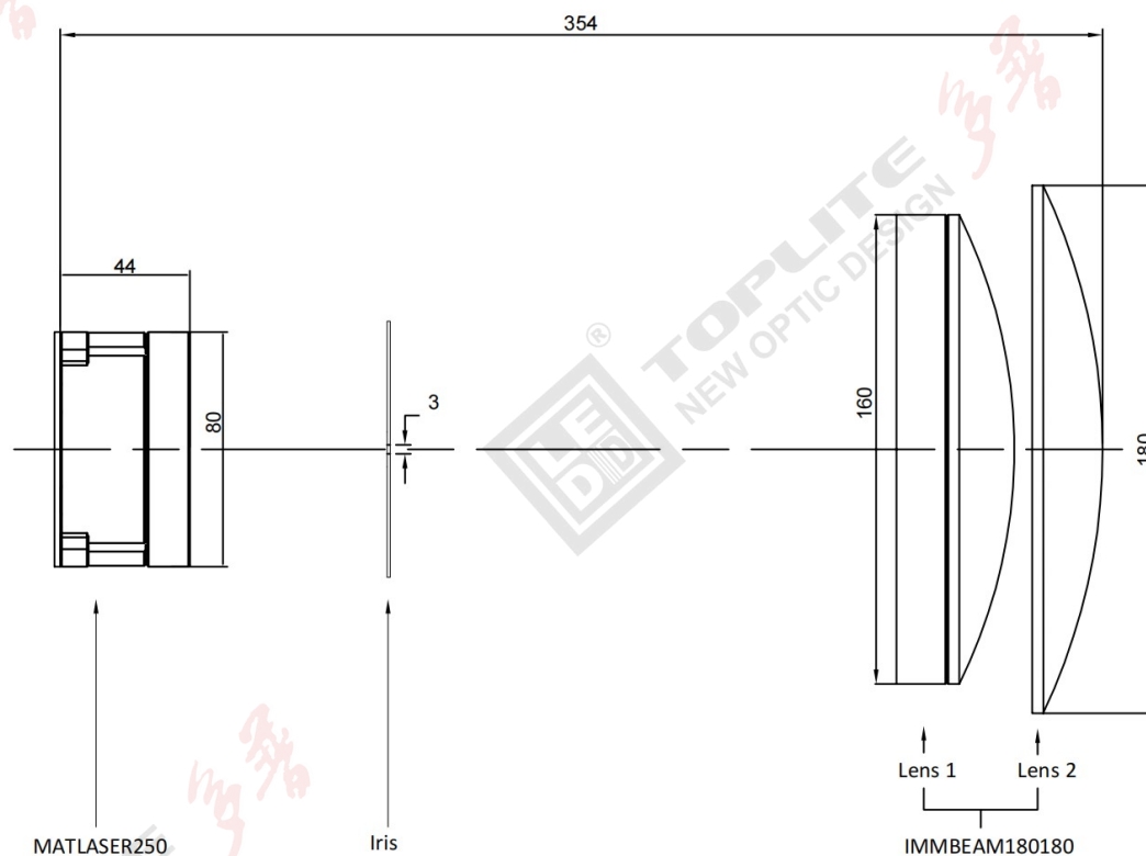
图 4: MAT Laser250 和 IMMBEAM180180 光路图
