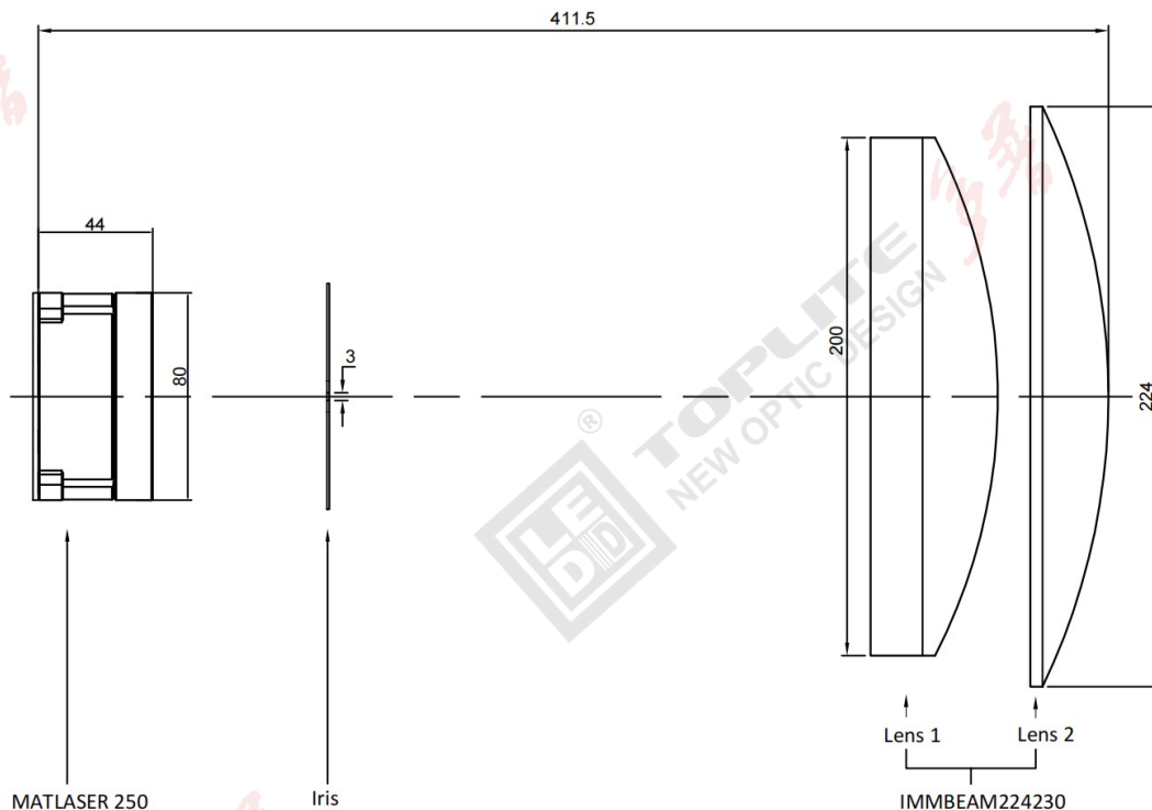
图 5: MAT Laser250 和 IMMBEAM224230 光路图
