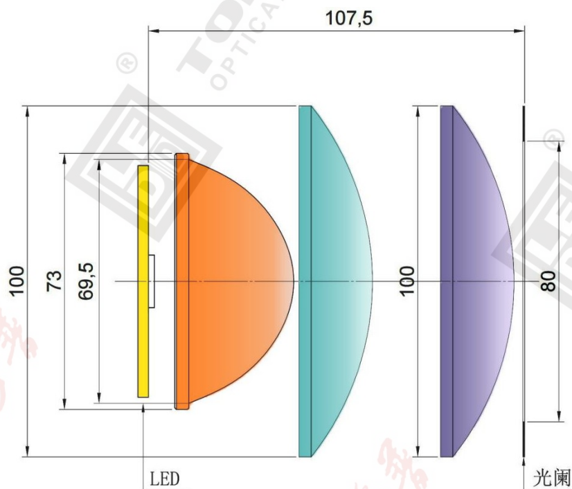
图：聚光透镜组可选项 IMMDX100X273 光路，聚光长度 E 为 107.5mm
