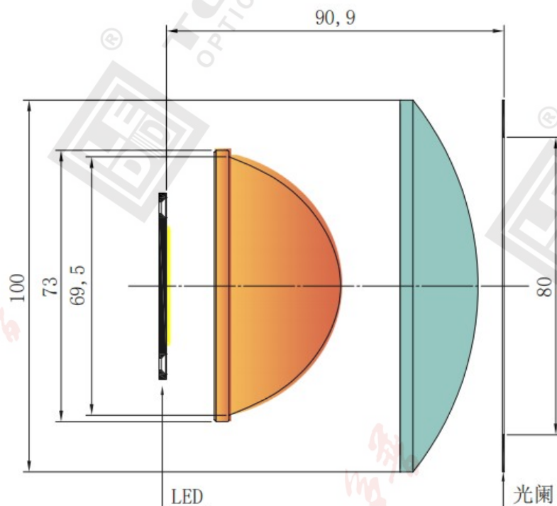
图：聚光透镜组可选项 IMMDX10073（高效率）光路，聚光长度 E 为 90.9mm
