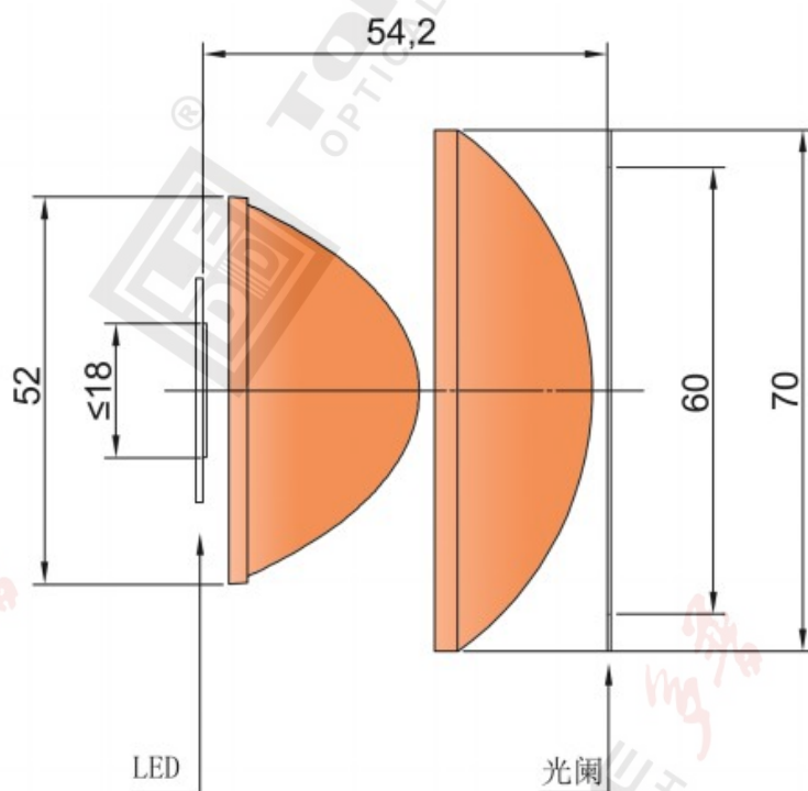
图：聚光透镜组可选项 IMMDX5270 光路，聚光长度 E 为 54.2mm,适合发光面 \leq\varnothing 18\text{mm} 的光源
